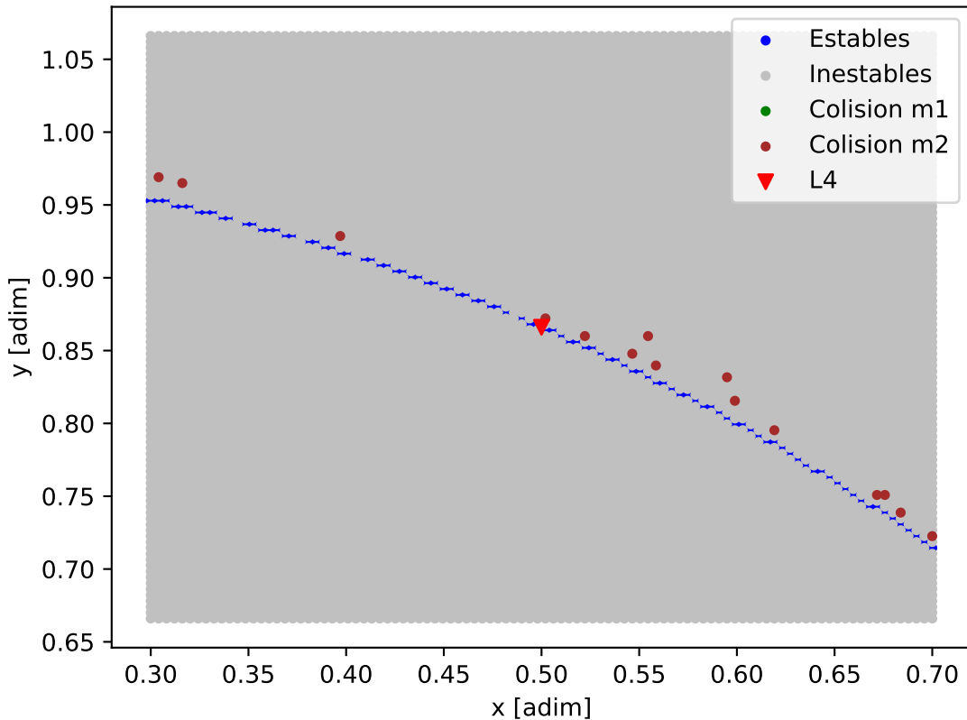
Mapa de estabilidad - K2-138
