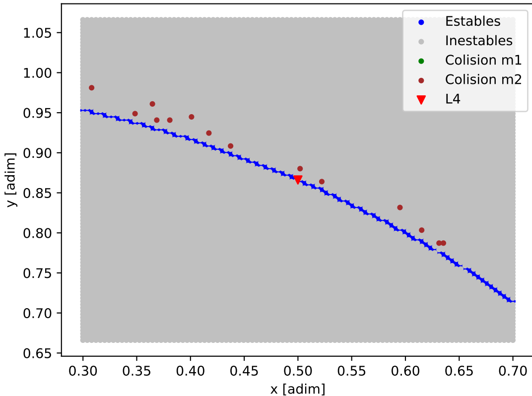
Mapa de estabilidad - WASP-47
