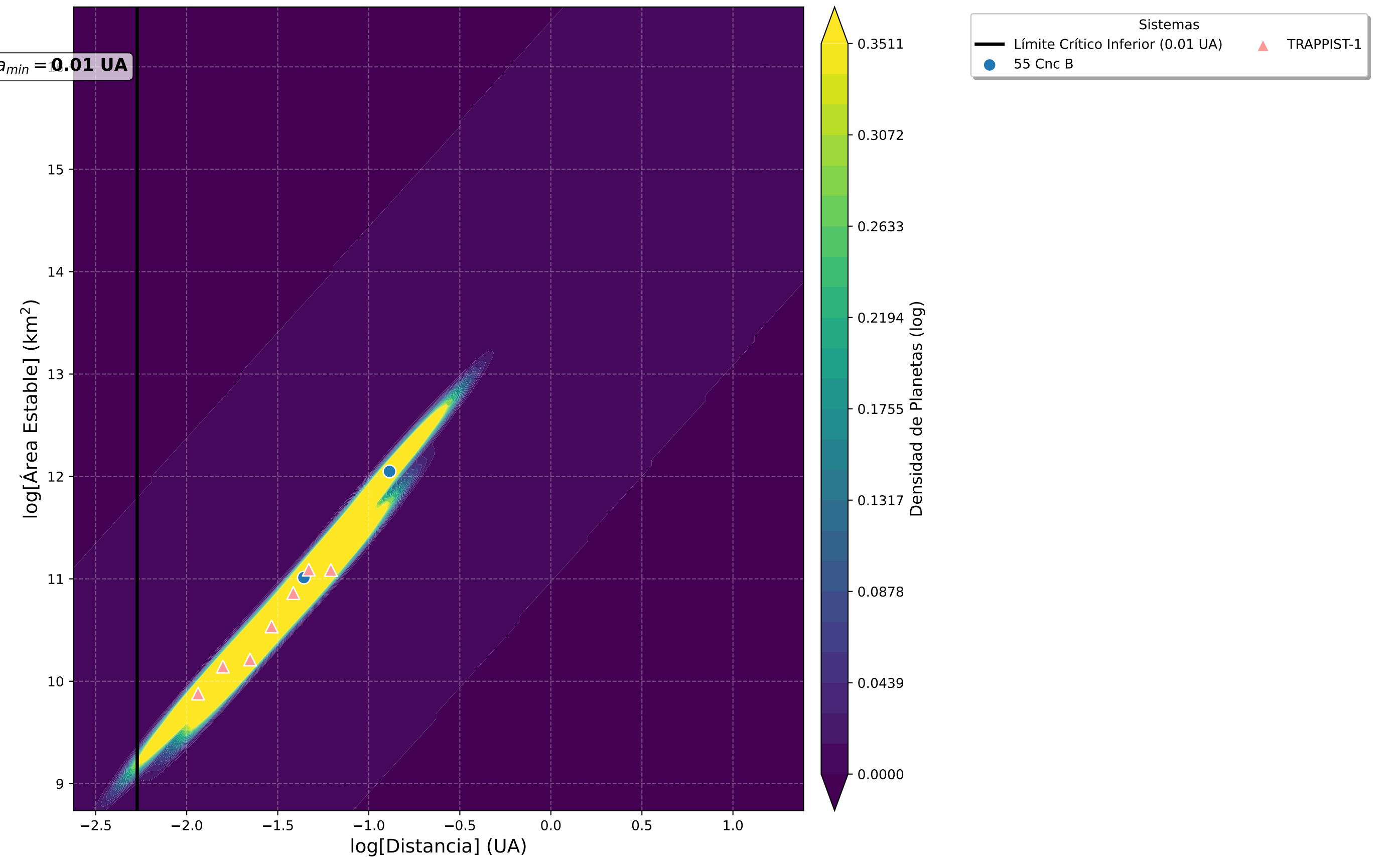
Sistemas con 7 planetas
