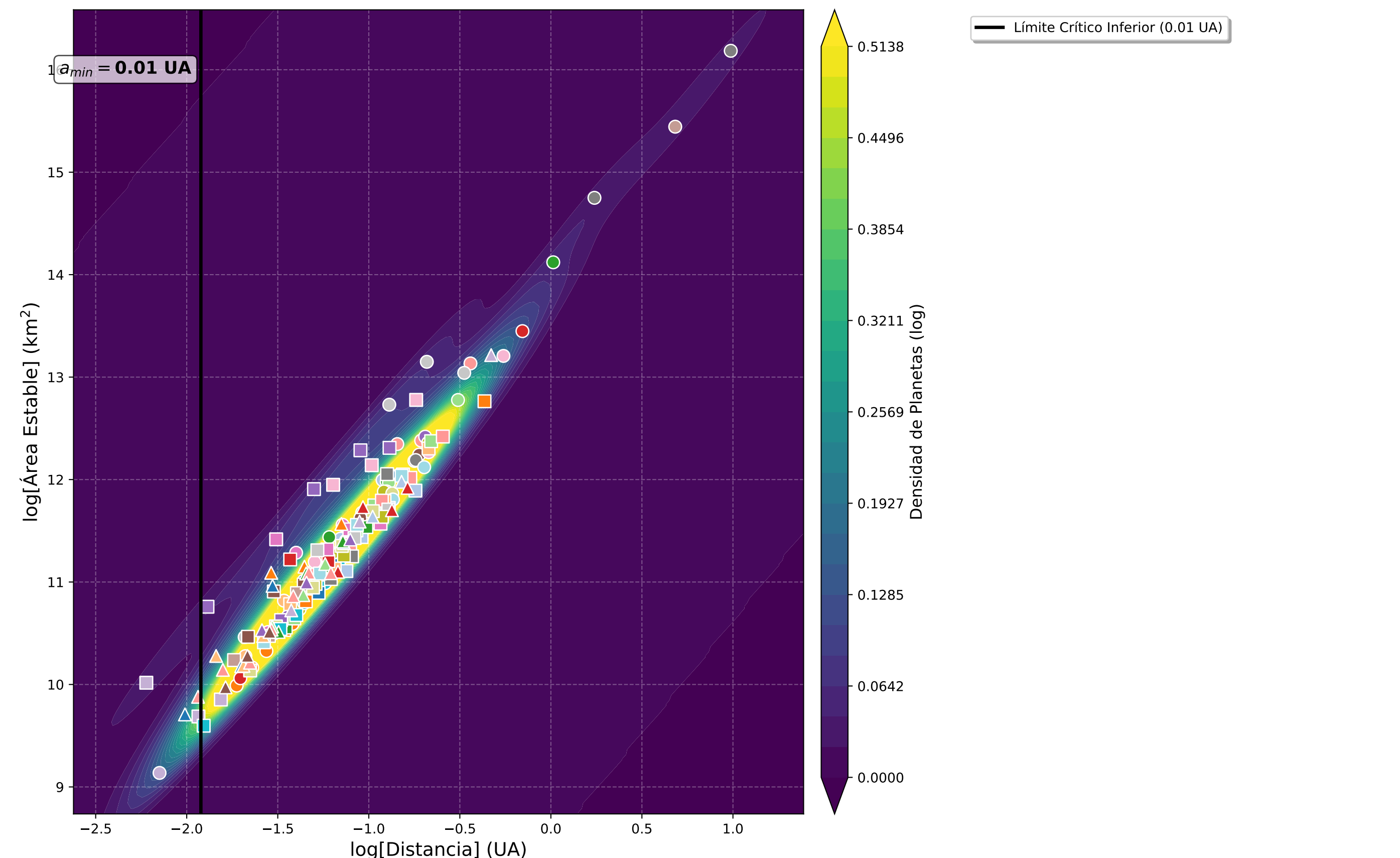
Sistemas con 3 planetas
