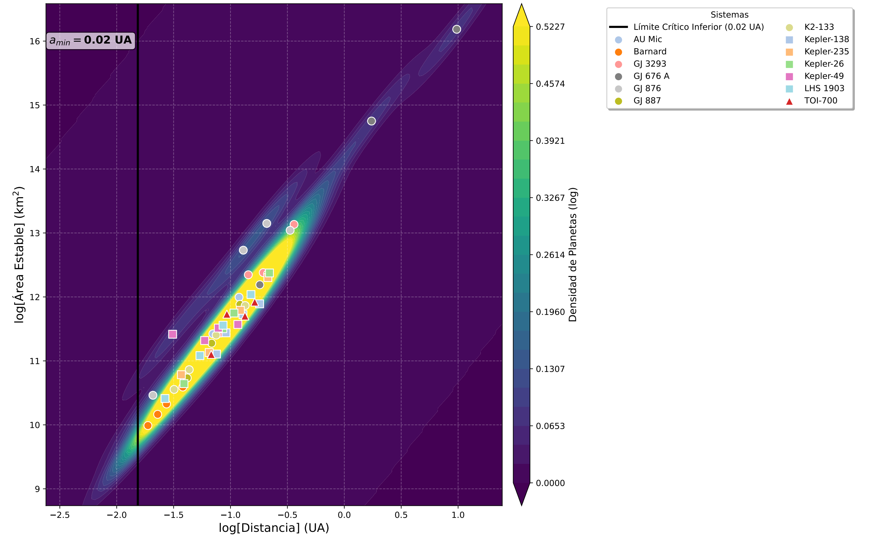
Sistemas con 5 planetas
