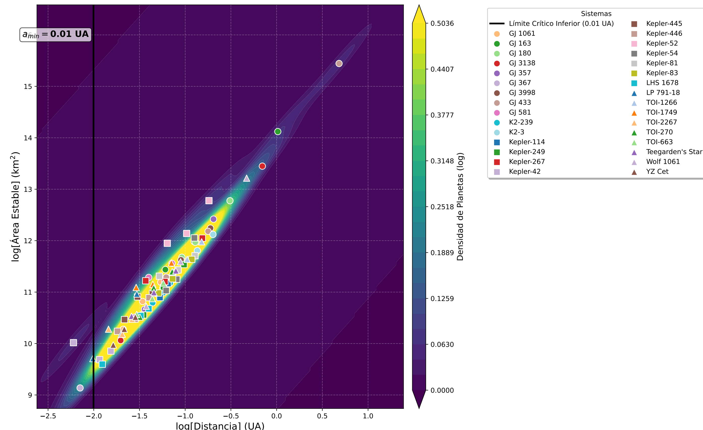
Sistemas con 4 planetas
