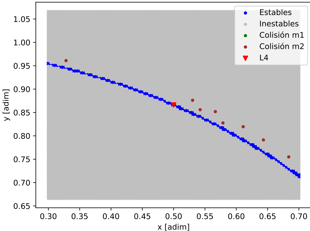
Mapa de estabilidad - HD_153557_HD_153557_b
