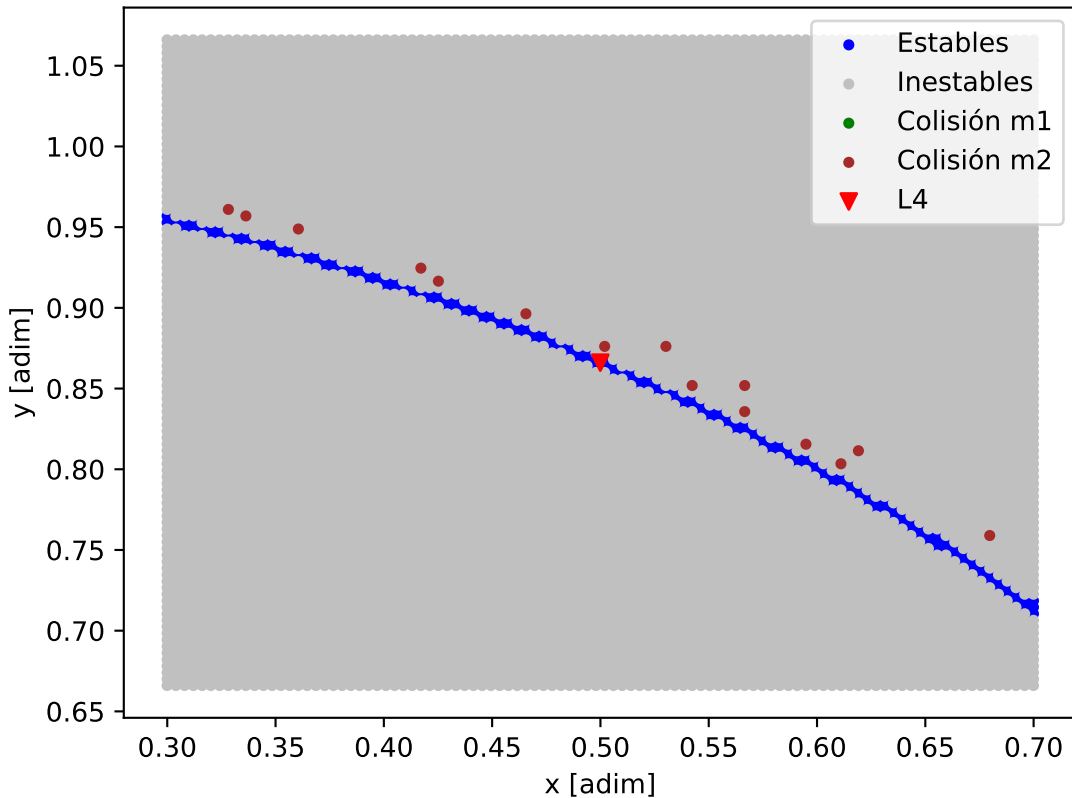
Mapa de estabilidad - HD_153557_HD_153557_c
