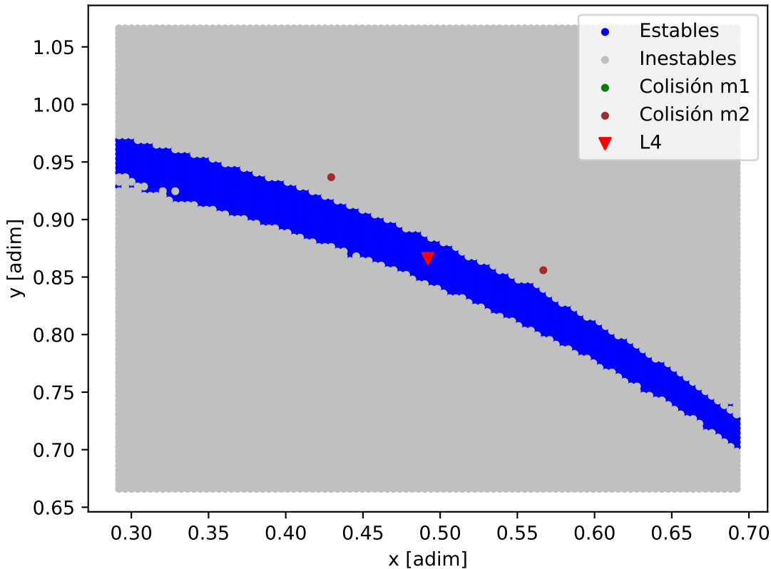
Mapa de estabilidad - HD_176986_HD_176986_c
