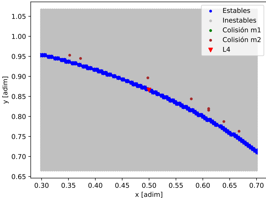
Mapa de estabilidad - HD_184010_HD_184010_b
