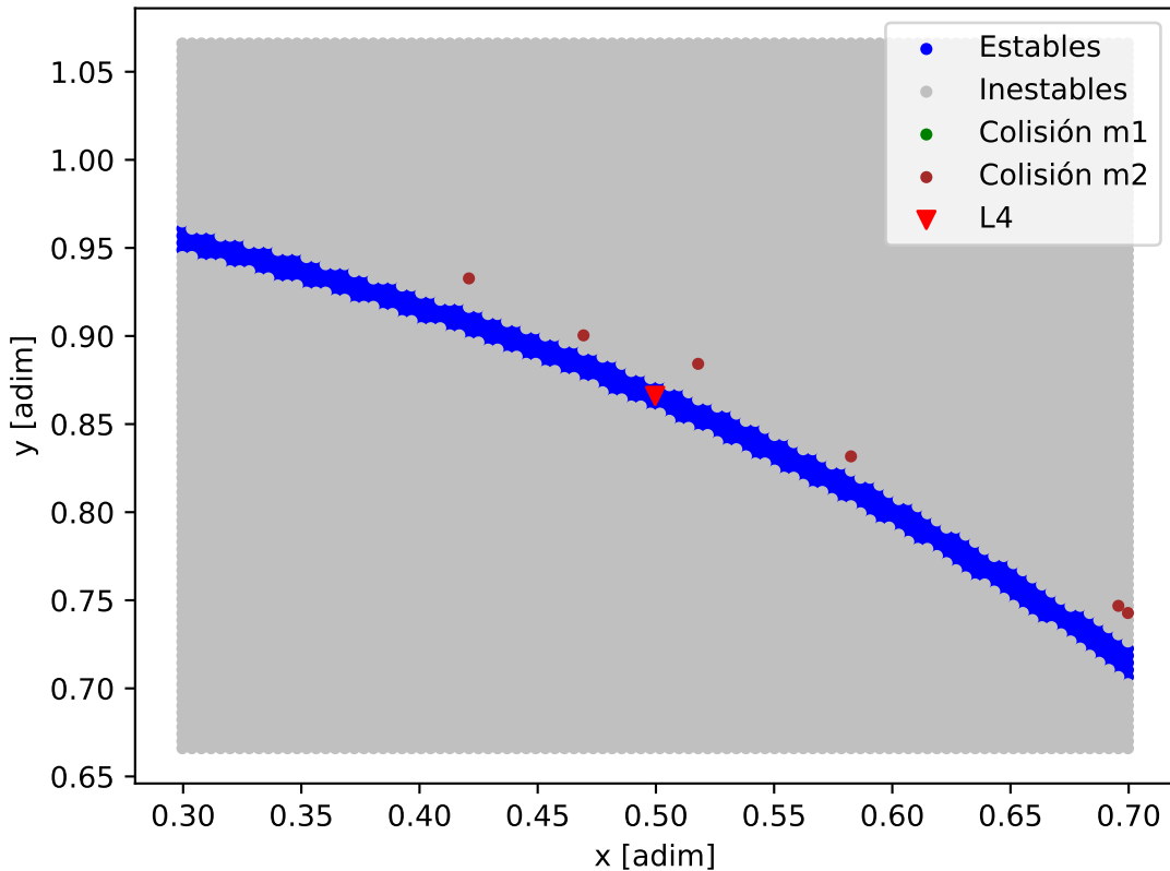
Mapa de estabilidad - HD_184010_HD_184010_d
