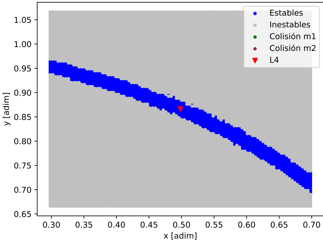
Mapa de estabilidad - HD_215152_HD_215152_c
