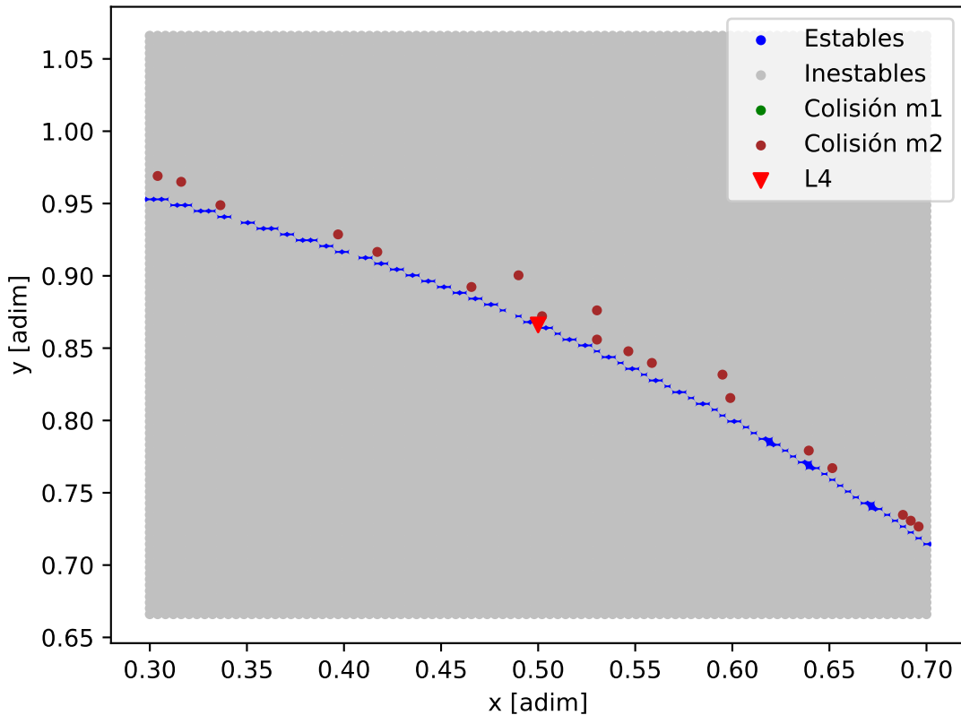
Mapa de estabilidad - HD_219134_HD_219134_c
