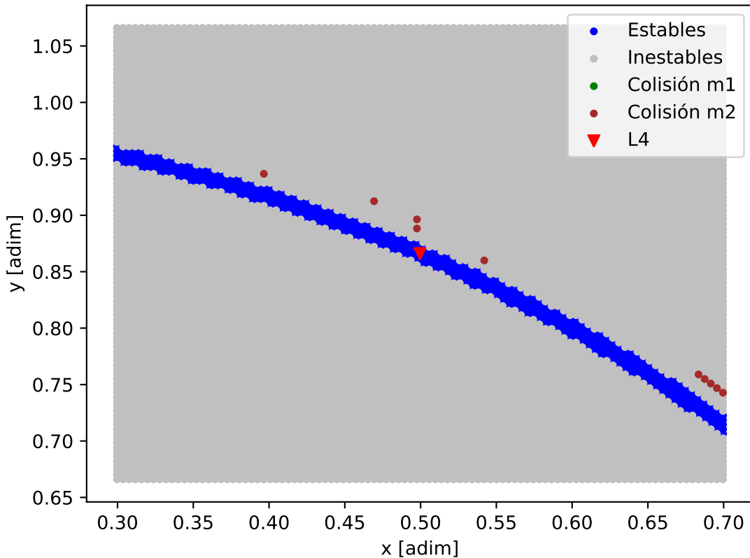
Mapa de estabilidad - HD_219134_HD_219134_h
