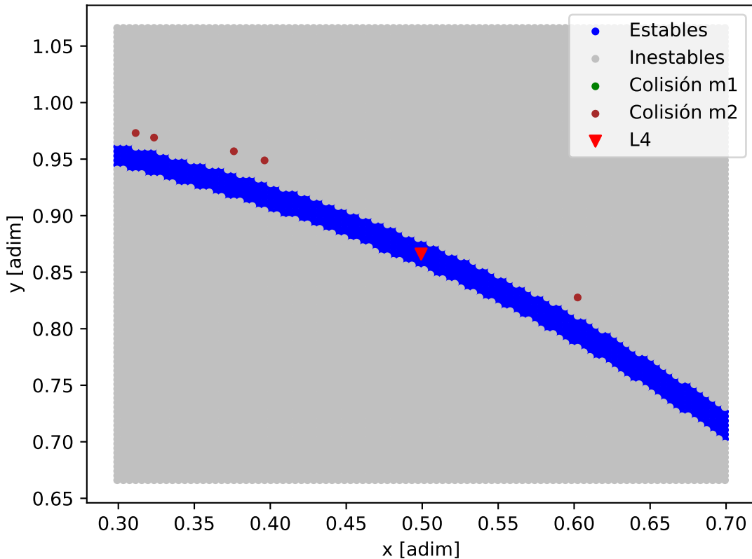
Mapa de estabilidad - HD_27894_HD_27894_b
