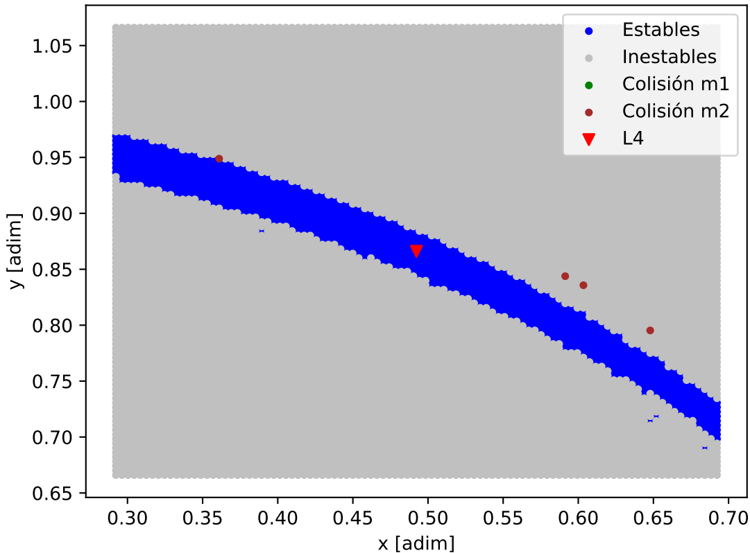
Mapa de estabilidad - HD_27894_HD_27894_d
