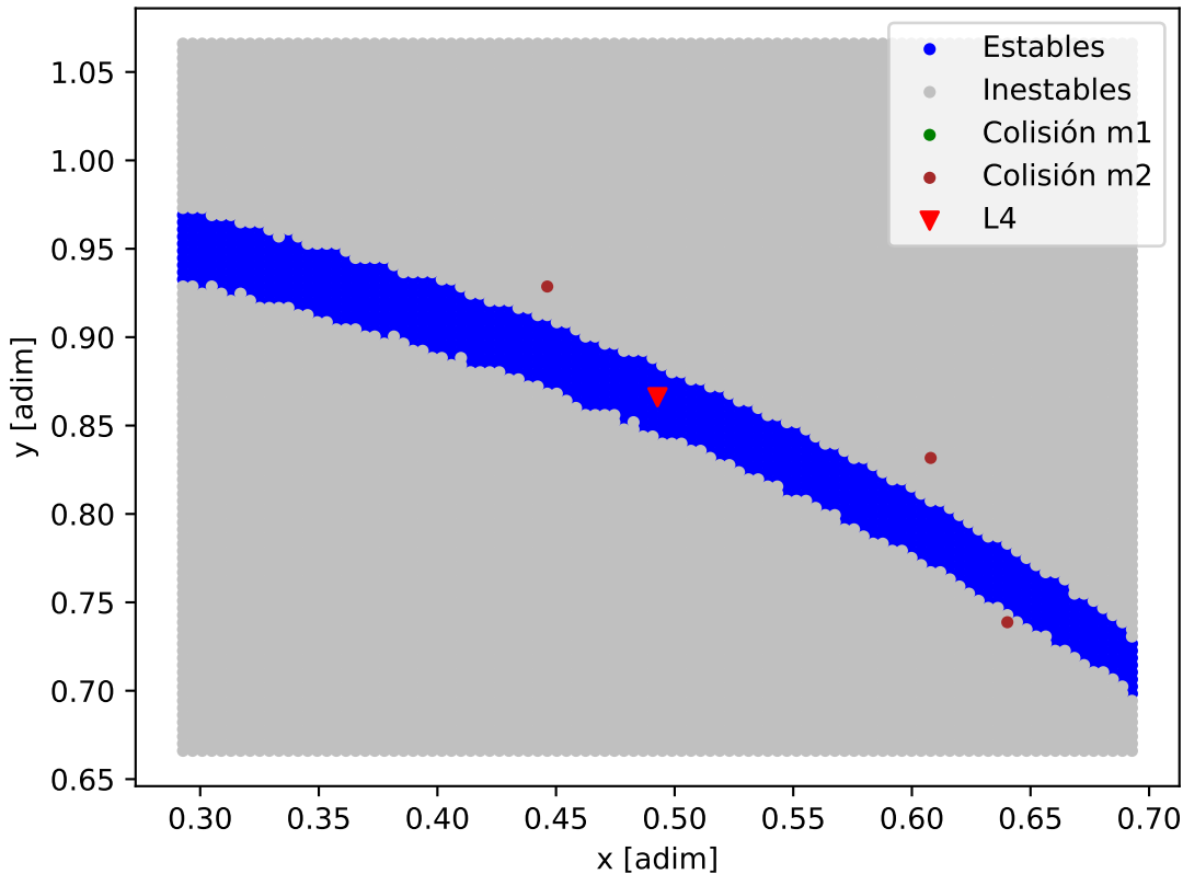
Mapa de estabilidad - HD_40307_HD_40307_c
