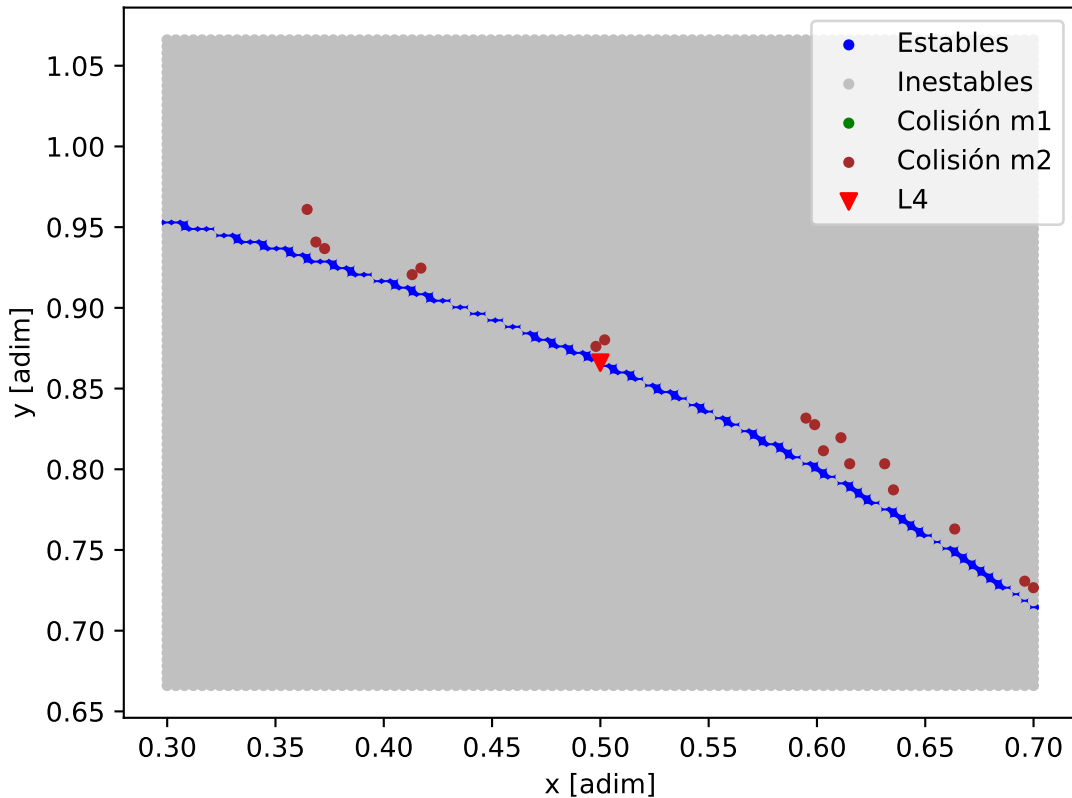
Mapa de estabilidad - HD_69830_HD_69830_b
