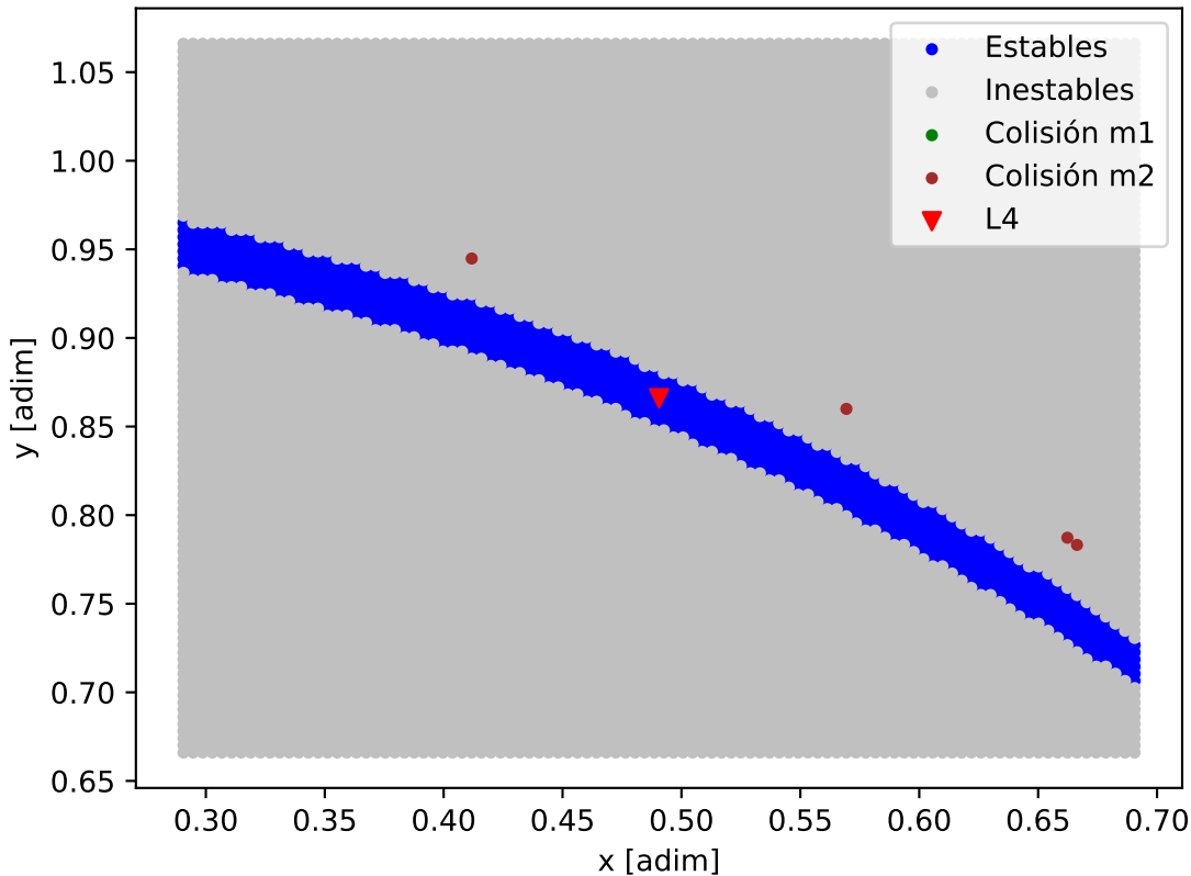
Mapa de estabilidad - HD_7924_HD_7924_b
