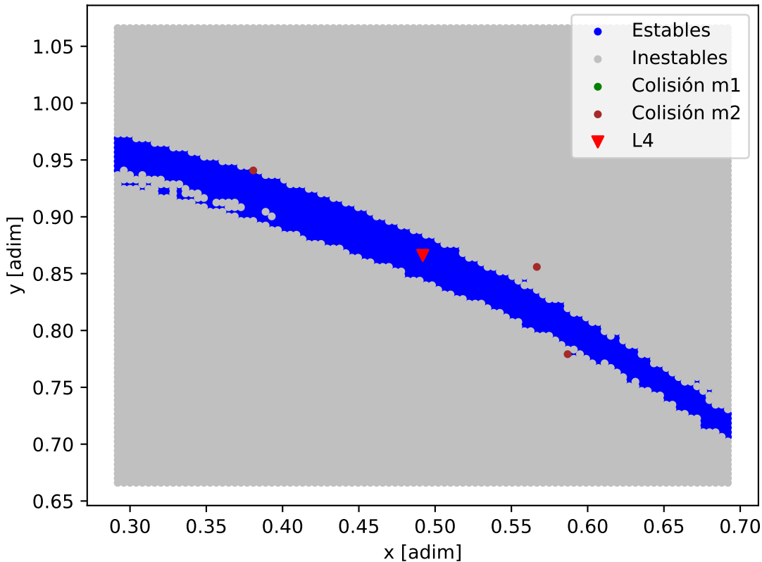
Mapa de estabilidad - HD_7924_HD_7924_c
