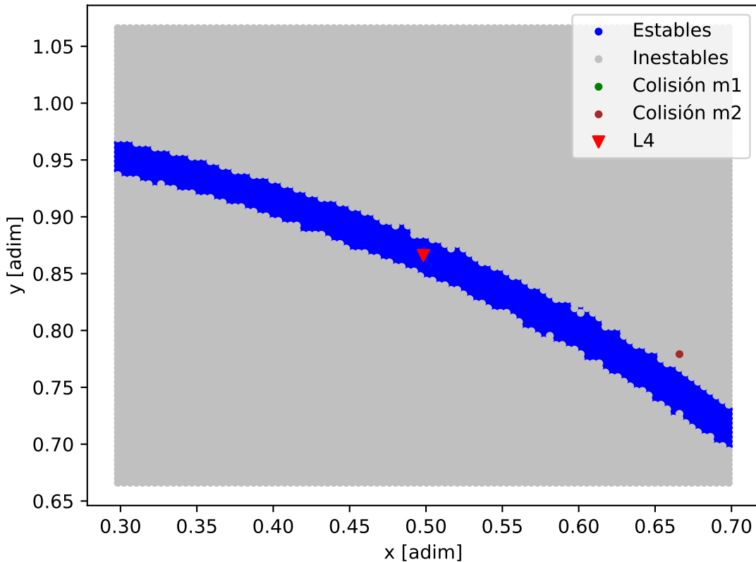
Mapa de estabilidad - HIP_57274_HIP_57274_d
