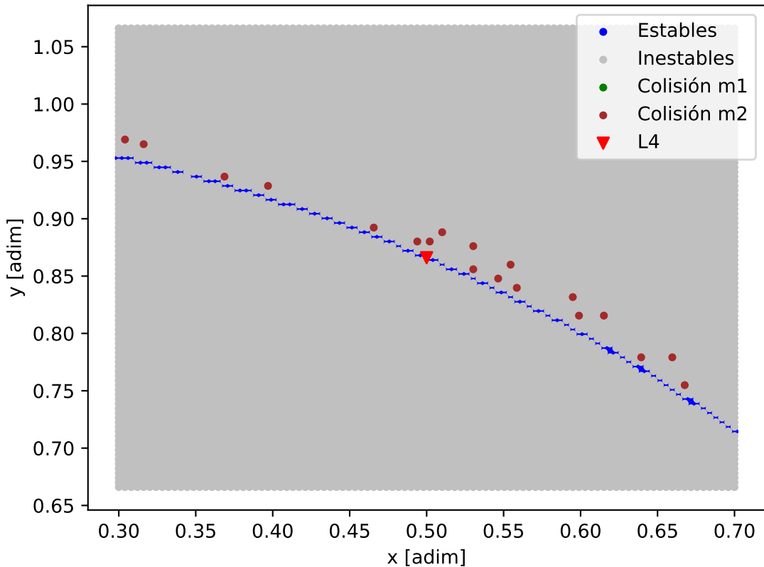
Mapa de estabilidad - K2-136_K2-136_b
