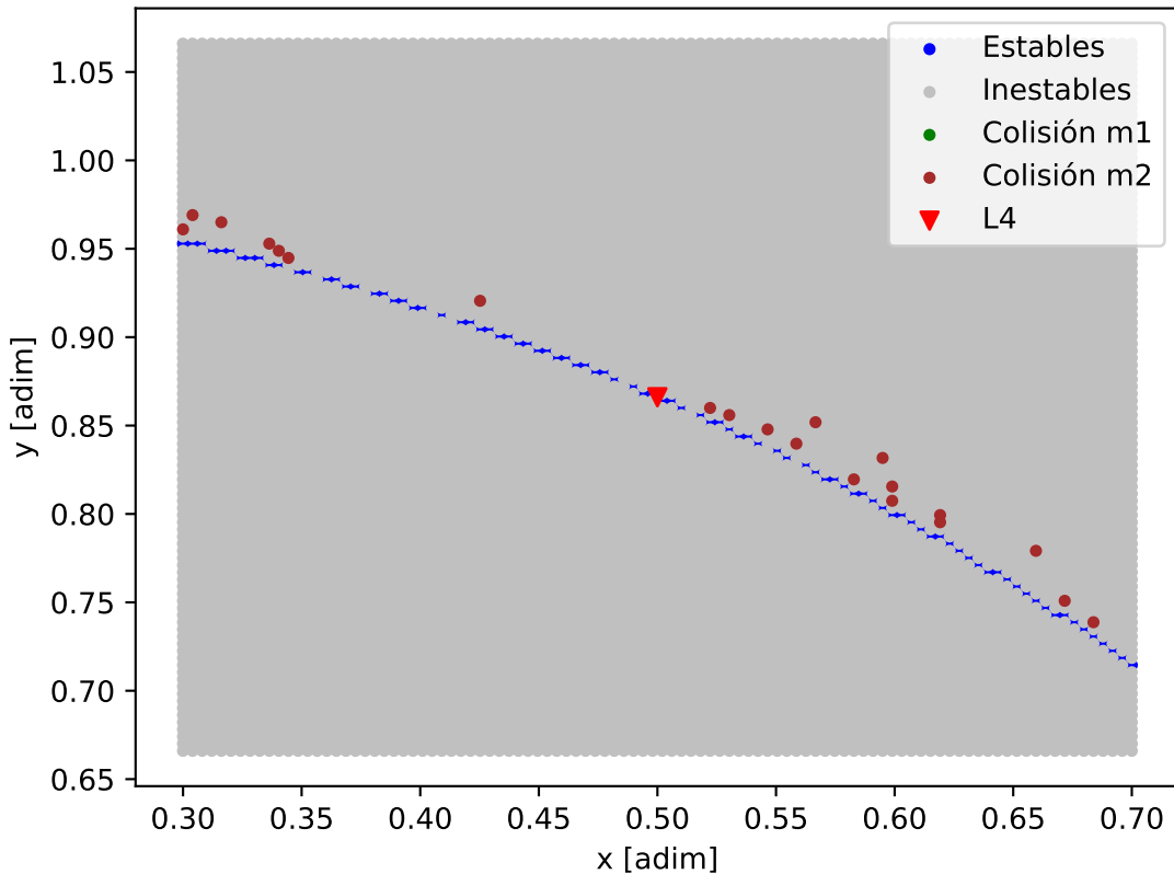
Mapa de estabilidad - K2-136_K2-136_d
