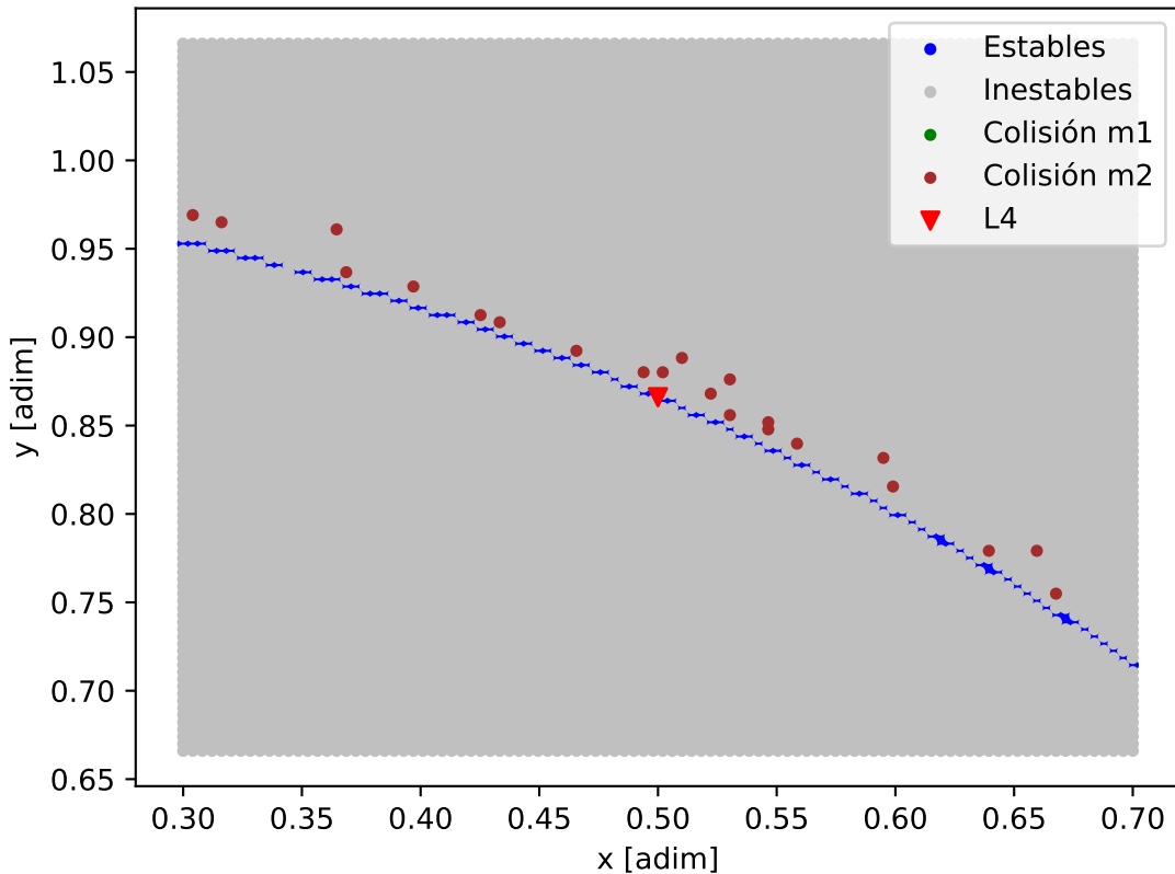
Mapa de estabilidad - K2-155_K2-155_b
