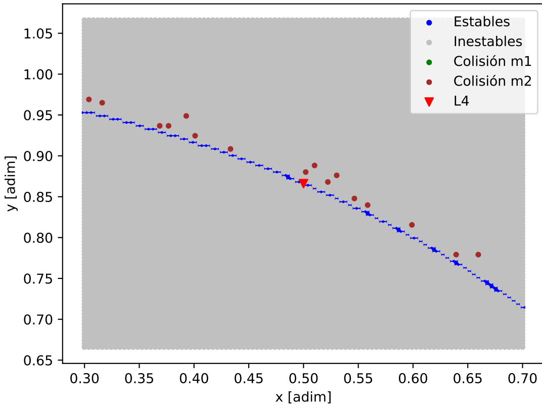
Mapa de estabilidad - K2-16_K2-16_b
