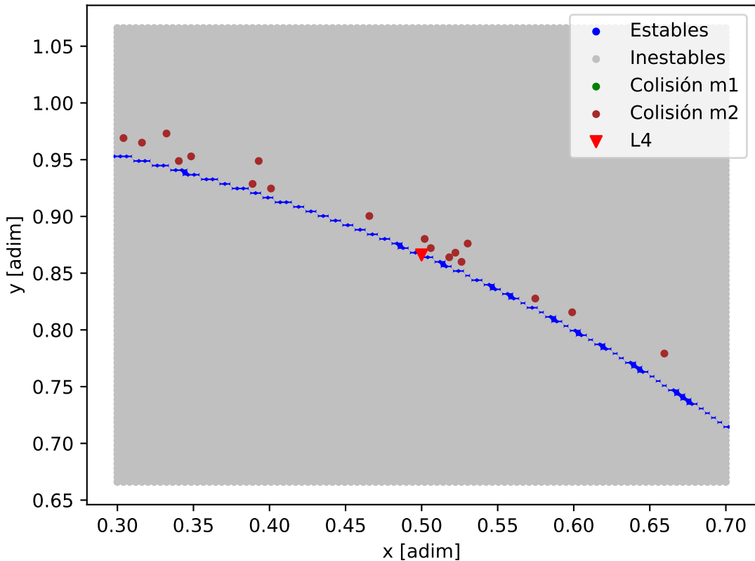
Mapa de estabilidad - K2-285_K2-285_d
