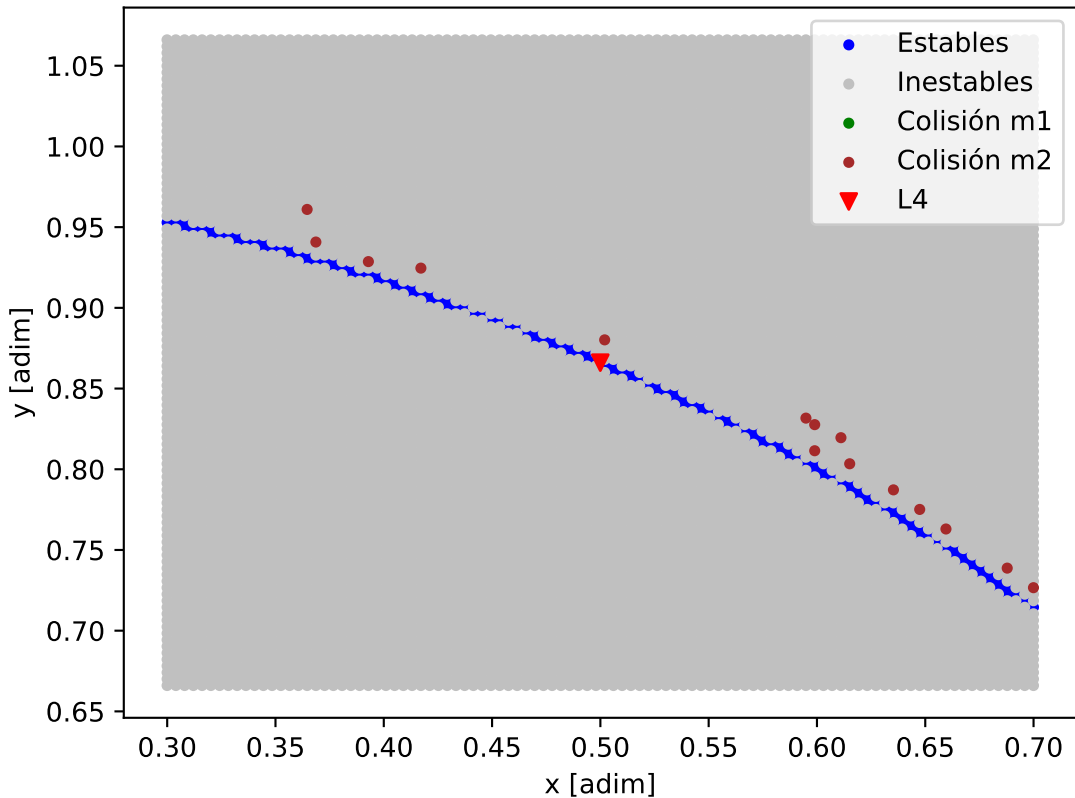
Mapa de estabilidad - K2-285_K2-285_e
