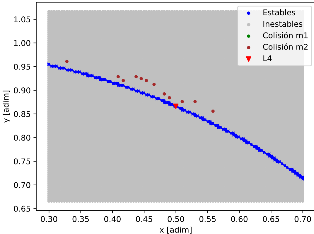
Mapa de estabilidad - Kepler-411_Kepler-411_c
