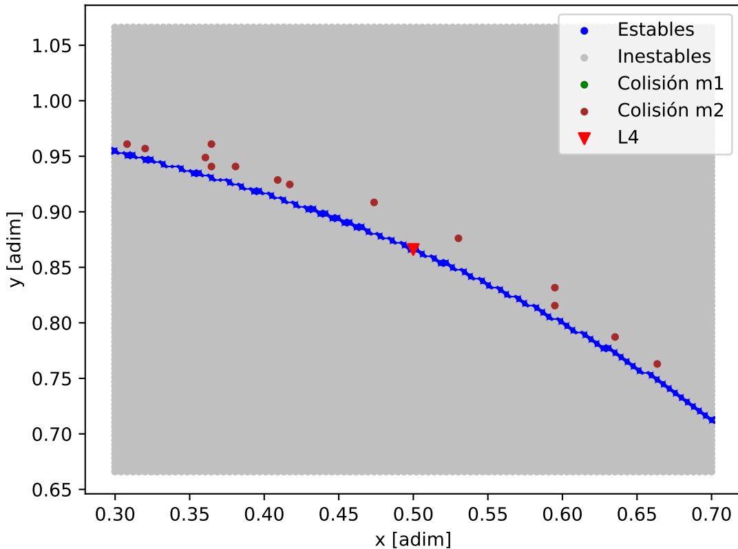
Mapa de estabilidad - Kepler-411_Kepler-411_d
