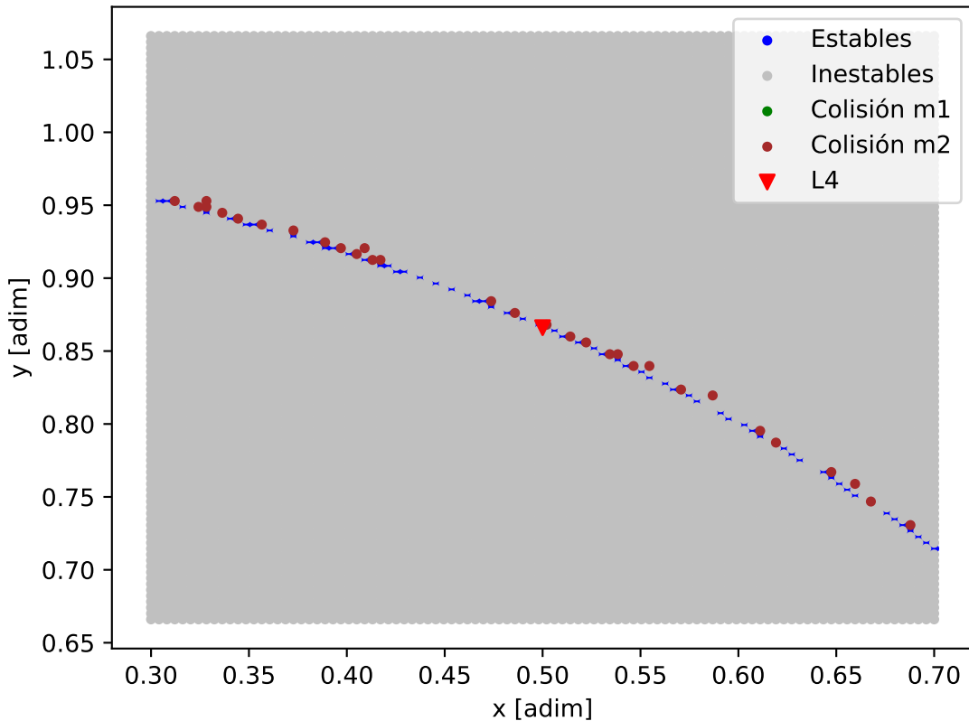
Mapa de estabilidad - Kepler-444_Kepler-444_c
