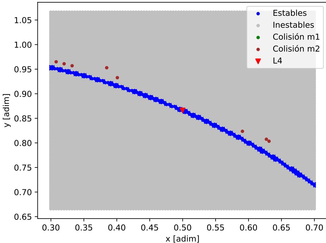
Mapa de estabilidad - Kepler-62_Kepler-62_f
