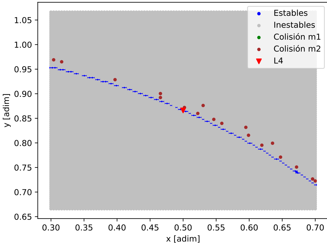
Mapa de estabilidad - Kepler-80_Kepler-80_e
