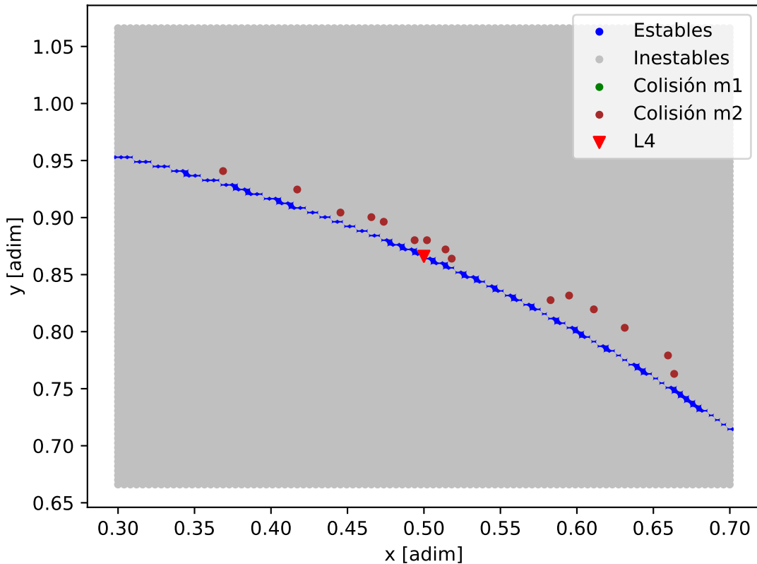
Mapa de estabilidad - TOI-1246_TOI-1246_c
