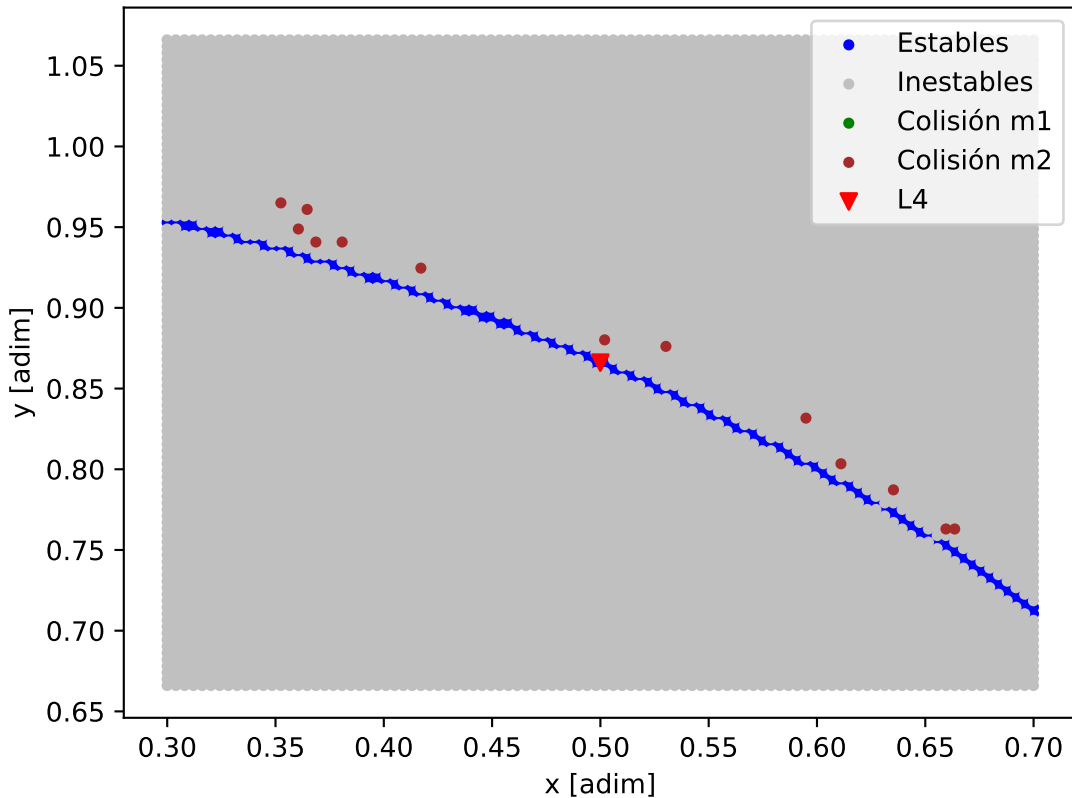
Mapa de estabilidad - TOI-1246_TOI-1246_e
