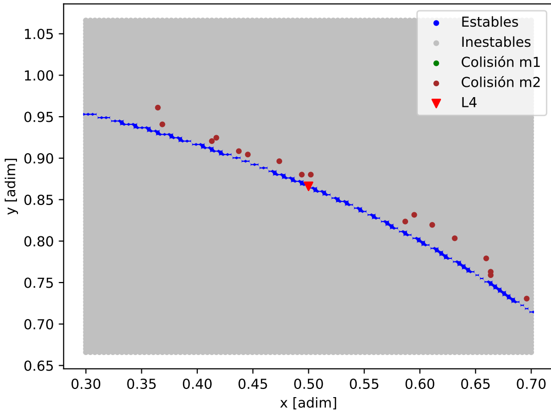
Mapa de estabilidad - TOI-125_TOI-125_b
