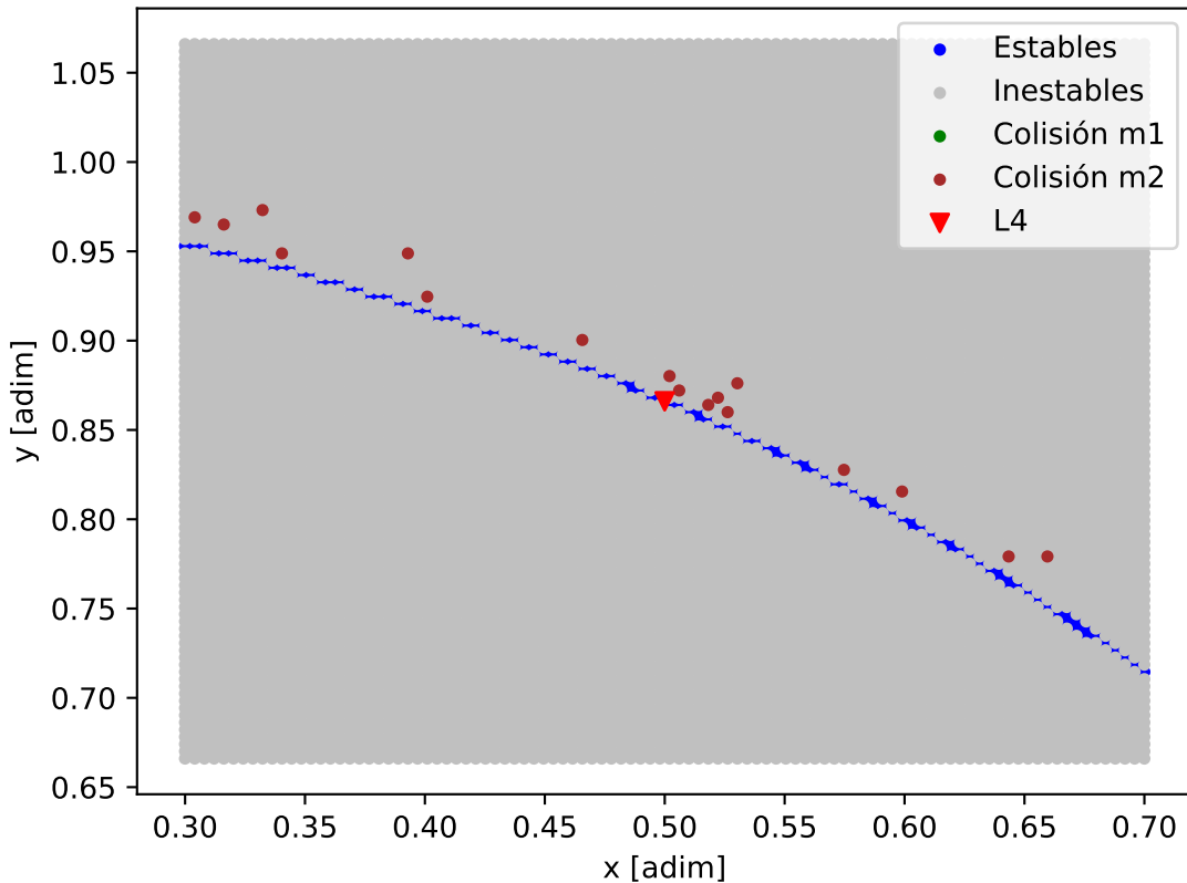
Mapa de estabilidad - TOI-125_TOI-125_c
