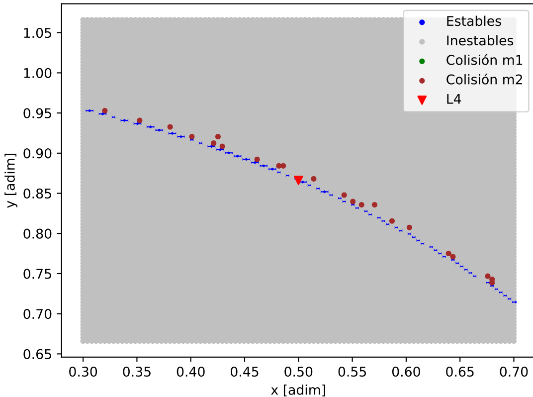
Mapa de estabilidad - TOI-178_TOI-178_b
