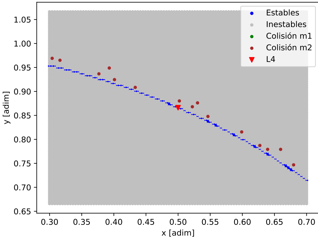
Mapa de estabilidad - TOI-178_TOI-178_c
