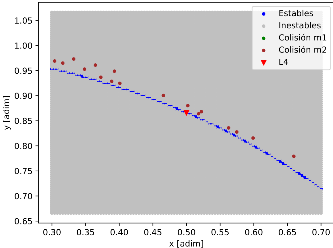
Mapa de estabilidad - TOI-178_TOI-178_d
