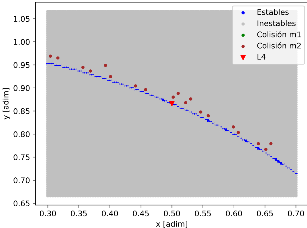
Mapa de estabilidad - TOI-178_TOI-178_g
