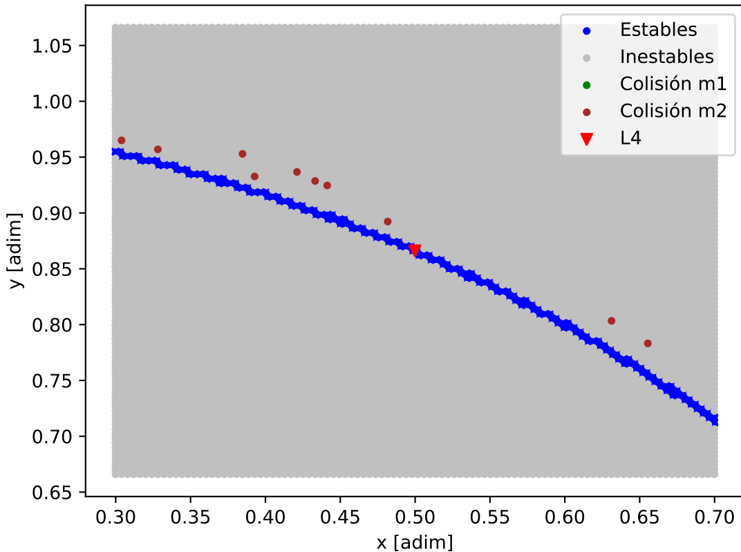
Mapa de estabilidad - TOI-4010_TOI-4010_d
