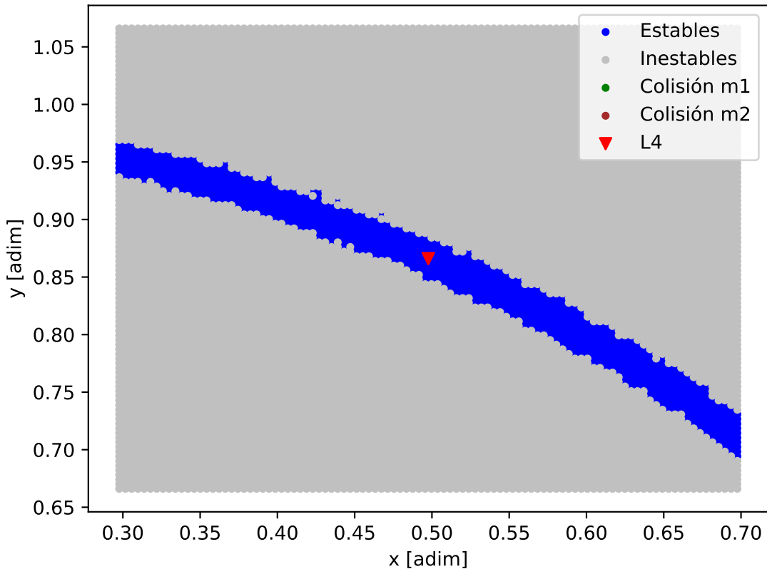
Mapa de estabilidad - TOI-4010_TOI-4010_e
