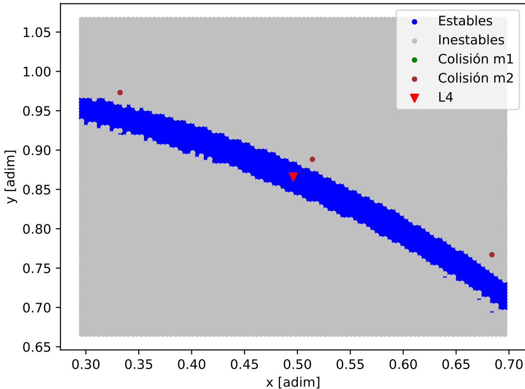
Mapa de estabilidad - TOI-4504_TOI-4504_c
