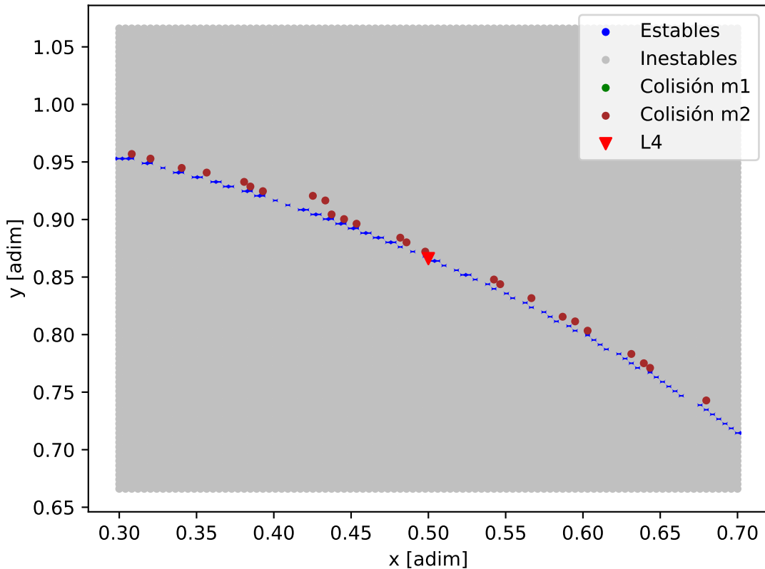
Mapa de estabilidad - TOI-500_TOI-500_b
