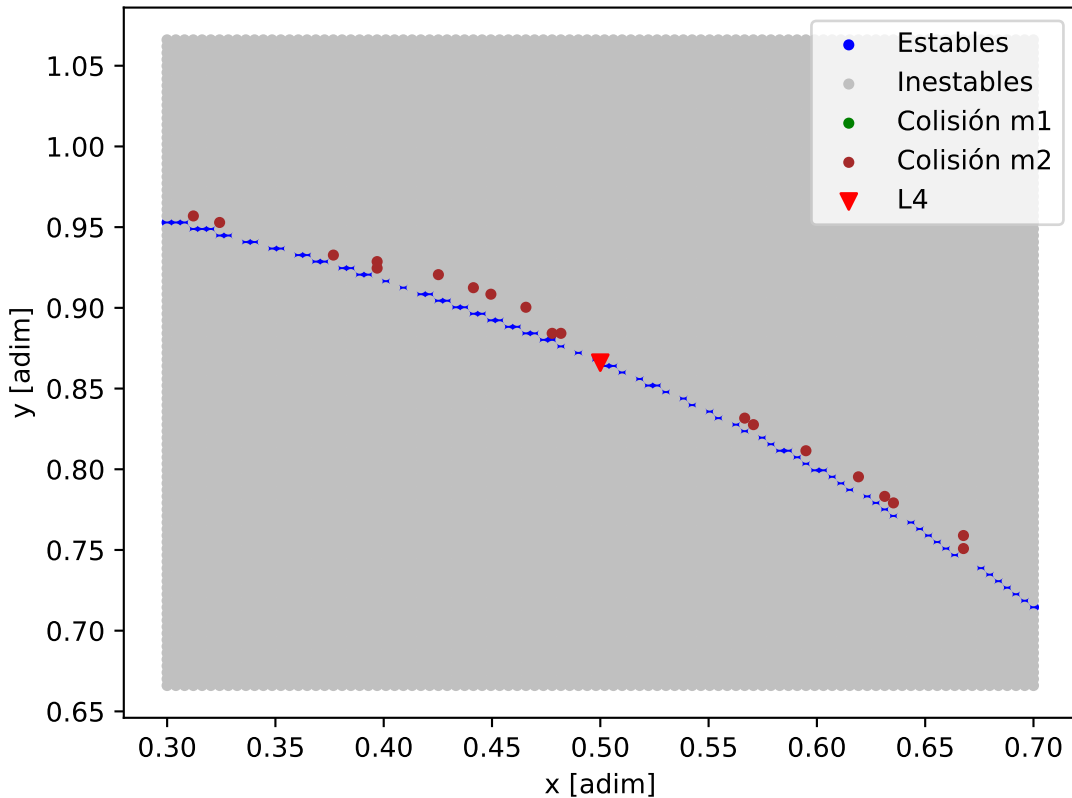
Mapa de estabilidad - TOI-5789_TOI-5789_b
