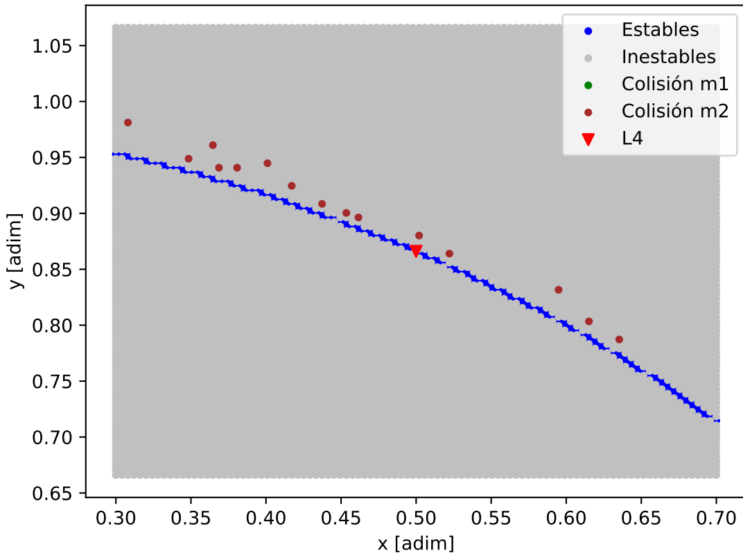
Mapa de estabilidad - TOI-5789_TOI-5789_e
