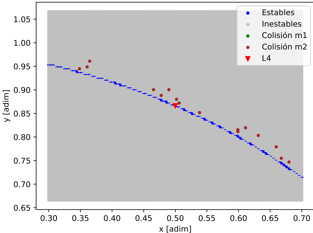
Mapa de estabilidad - TOI-712_TOI-712_d
