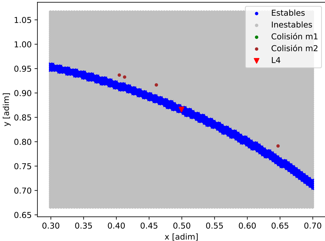
Mapa de estabilidad - WASP-132_WASP-132_b
