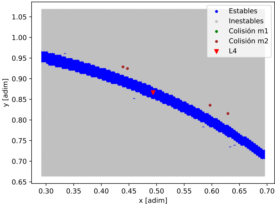
Mapa de estabilidad - WASP-132_WASP-132_d
