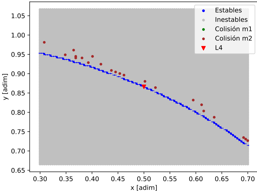
Mapa de estabilidad - DMPP-1_DMPP-1_b
