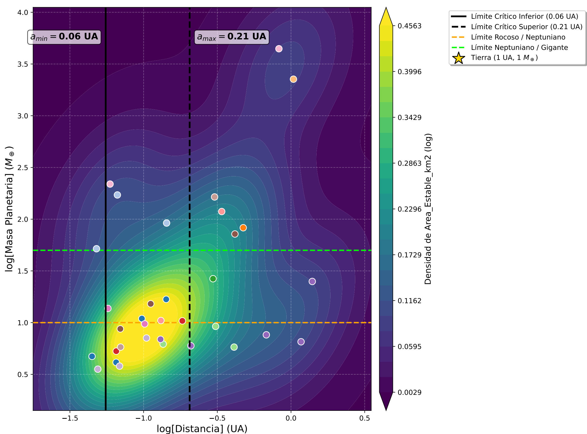
Sistemas con 0 planetas (Area_Estable_km2)
