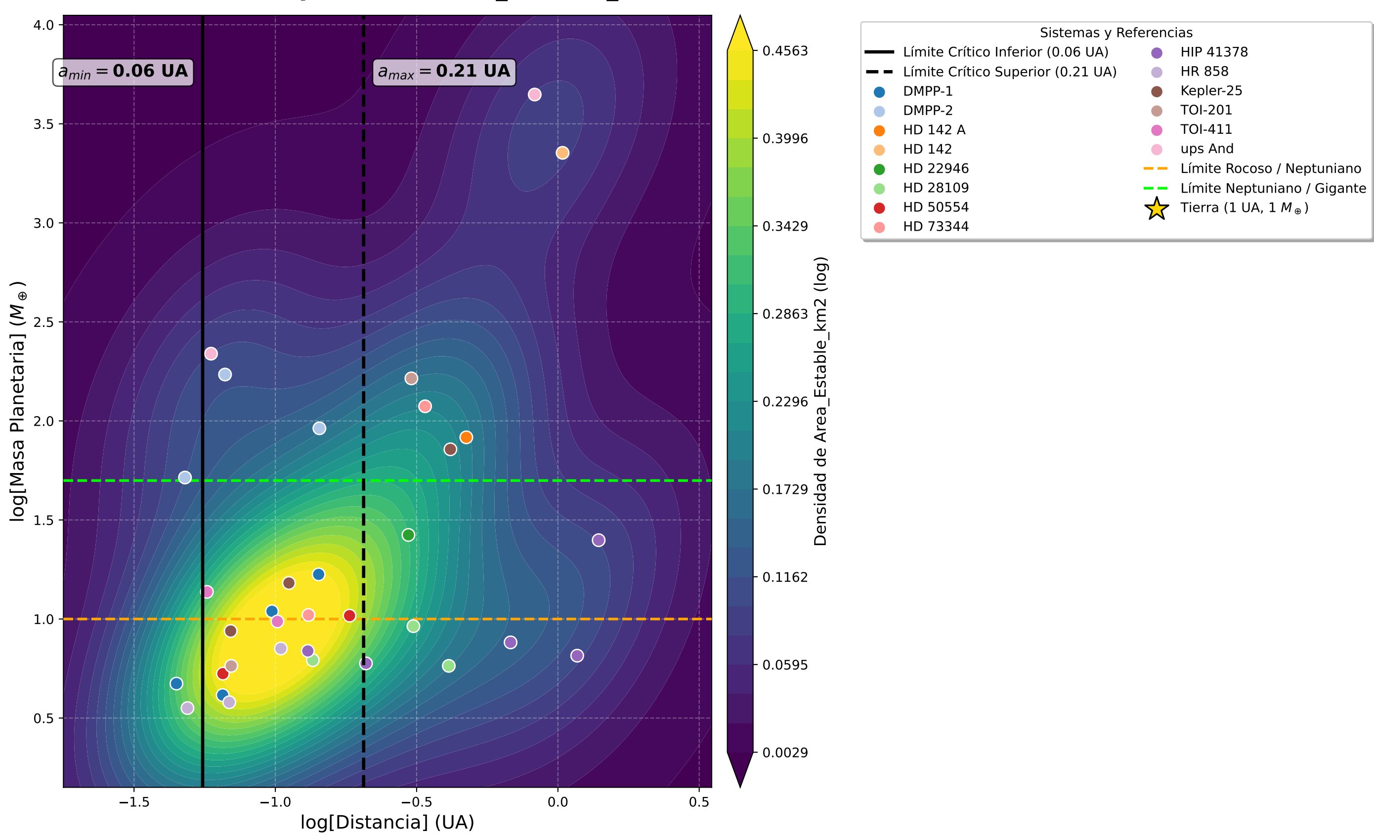
Sistemas con 0 planetas (Area_Estable_km2)
