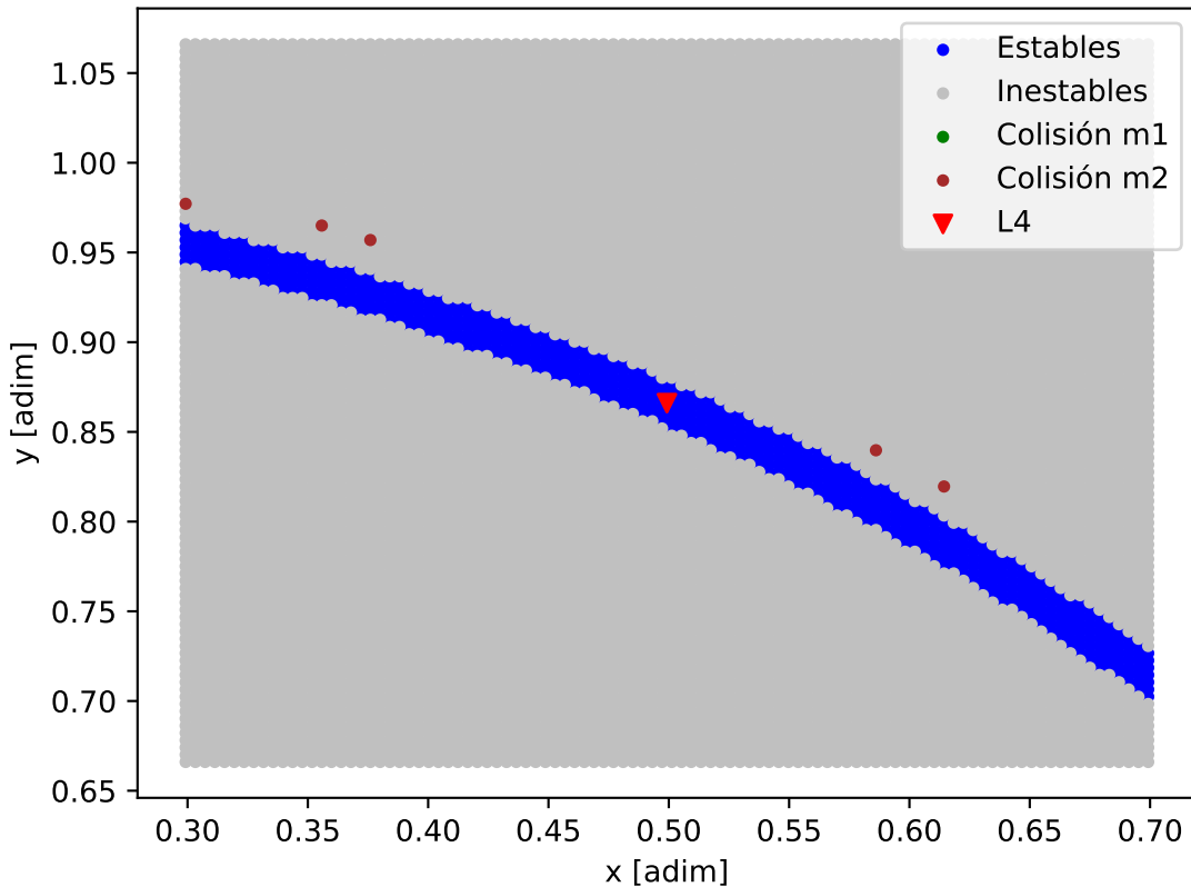
Mapa de estabilidad - 55_Cnc_55_Cnc_b
