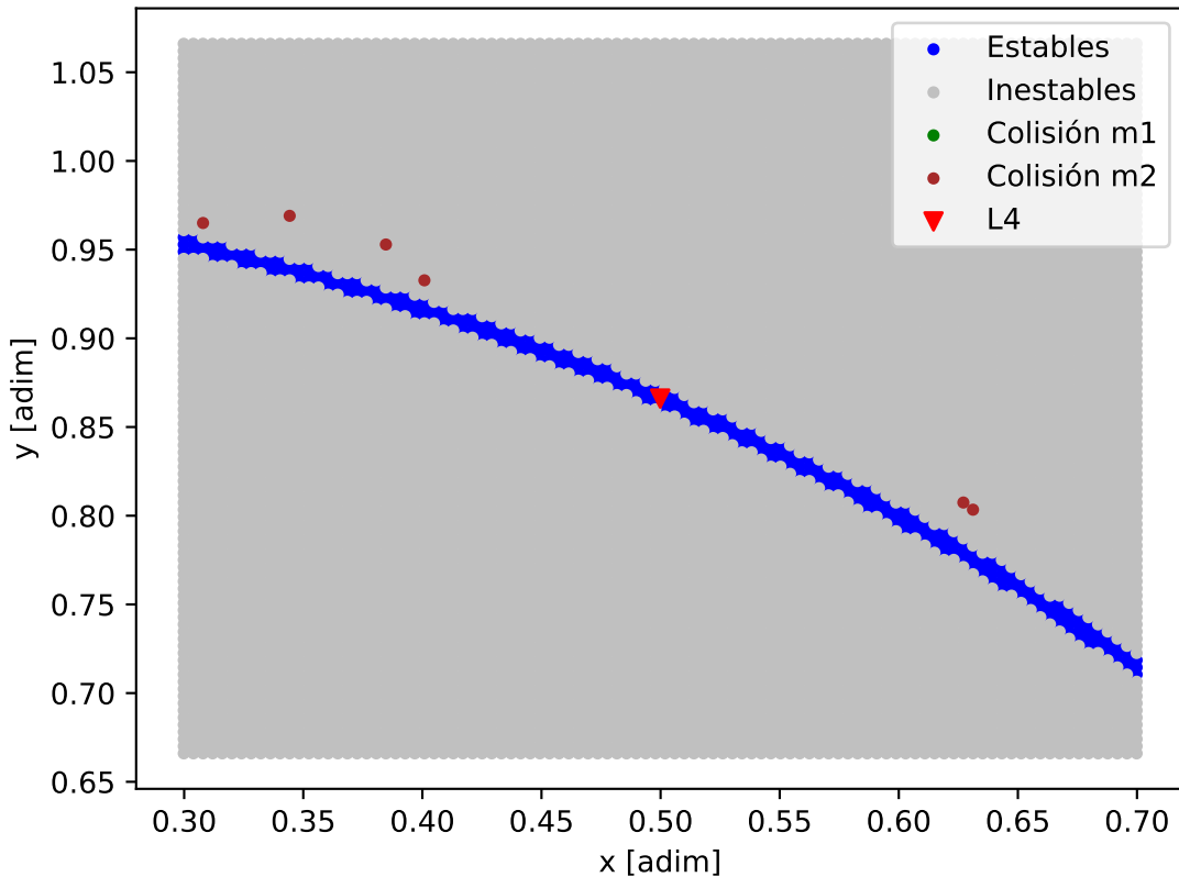
Mapa de estabilidad - 55_Cnc_55_Cnc_c
